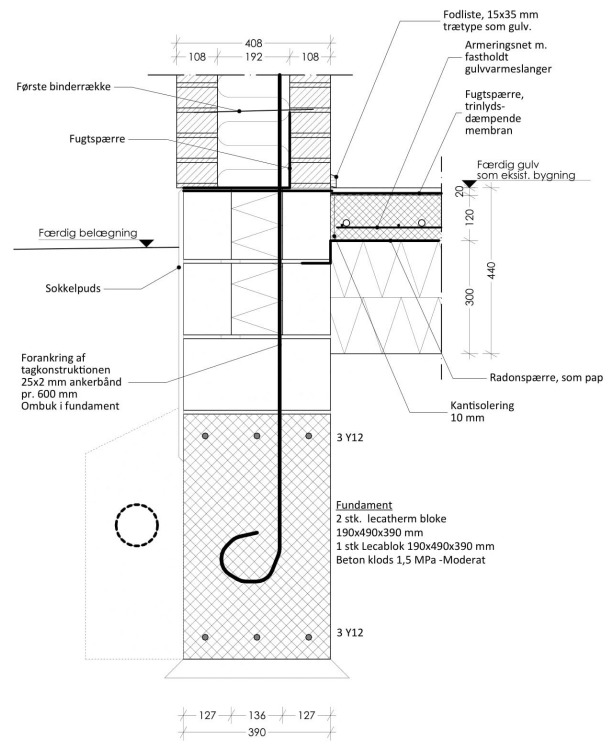
F-01 F-Detalje 1:10
