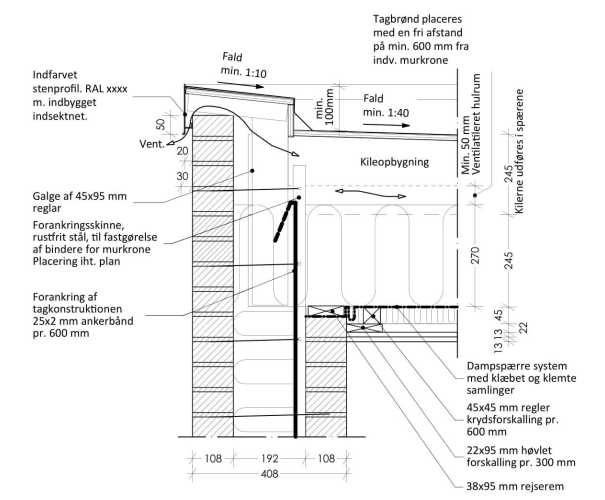
T-01 T-Detalje 1:10
