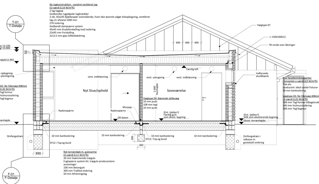
A-A Principsnit 1:50
